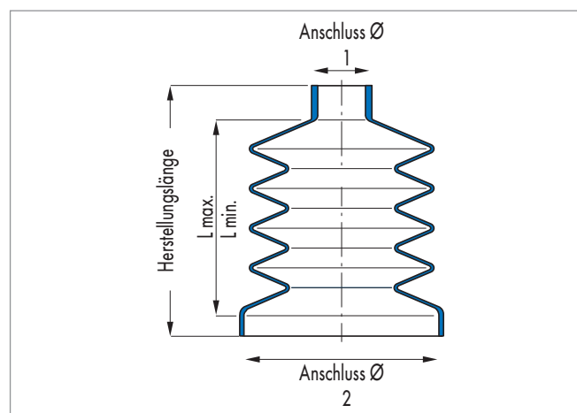
Maßskizze Mehrfaltenbalg
